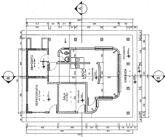
PLANTA REFORMA ESCALA 1:100
