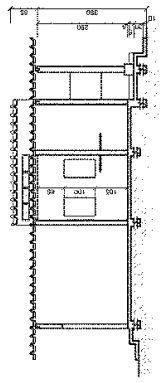
CORTE AA ESCALA 1:100
